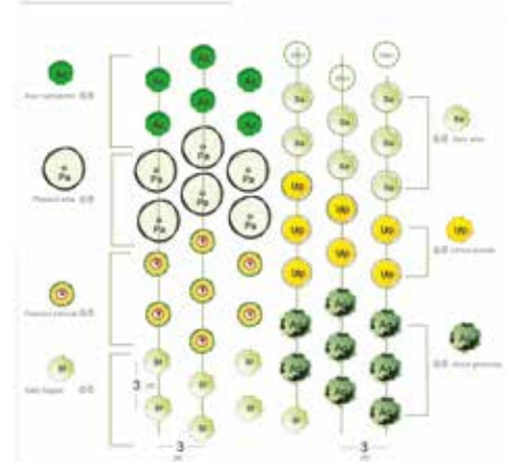
Schema di impianto della vegetazione, dal progetto esecutivo
