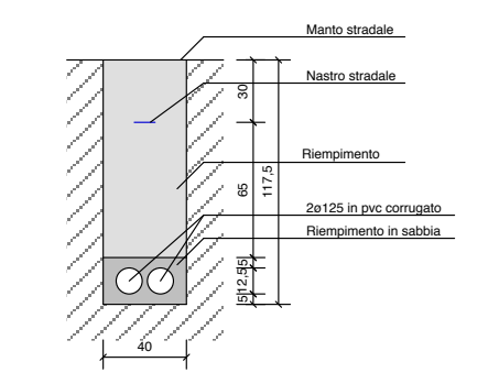
PARTICOLARE SEZIONE DI POSA Scala 1:20
